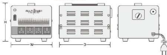
形状・寸法図 SU-1700G
