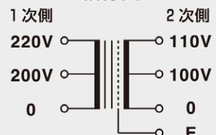
結線図
