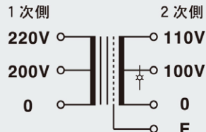
結線図
