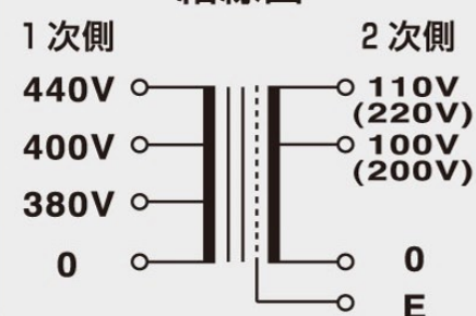
結線図
