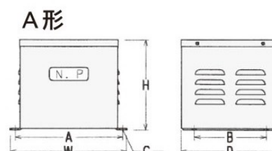
形状・寸法図
