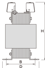
UP形（ねじアップ式端子台）
