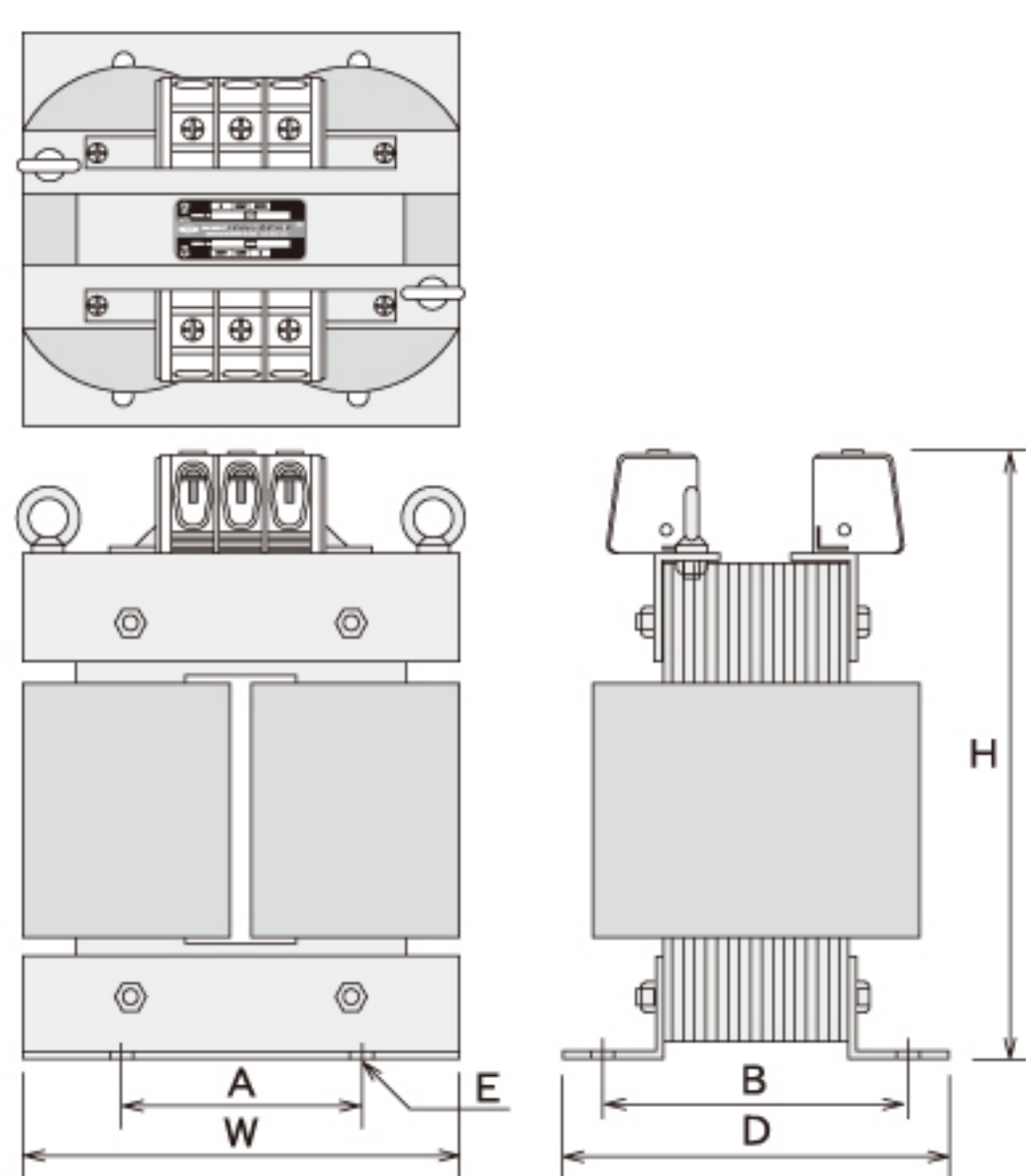
UP形（ねじアップ式端子台）
