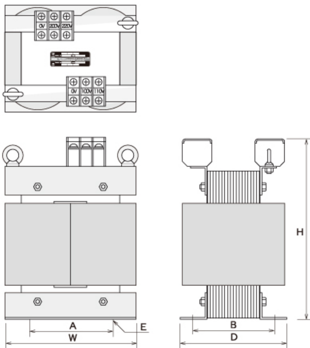
KT形（端子台）
