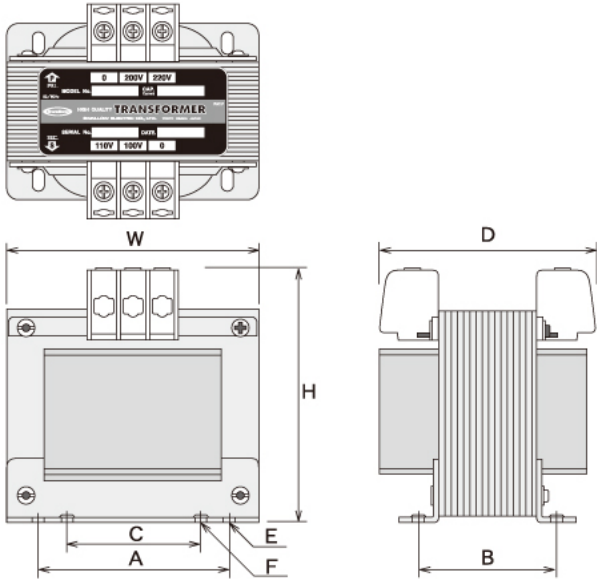
UP形（ねじアップ式端子台）
