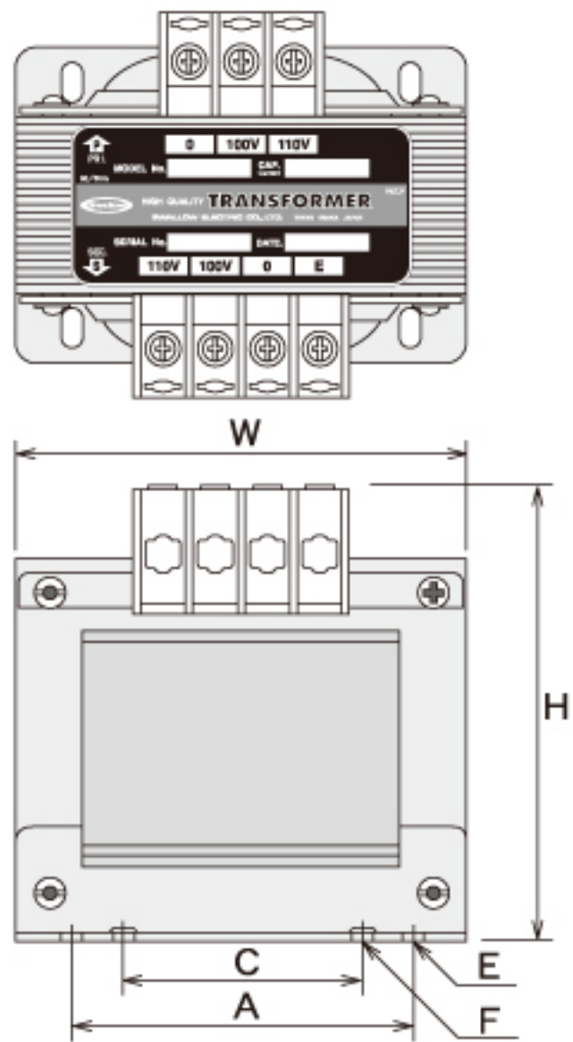
UP形（ねじアップ式端子台）
