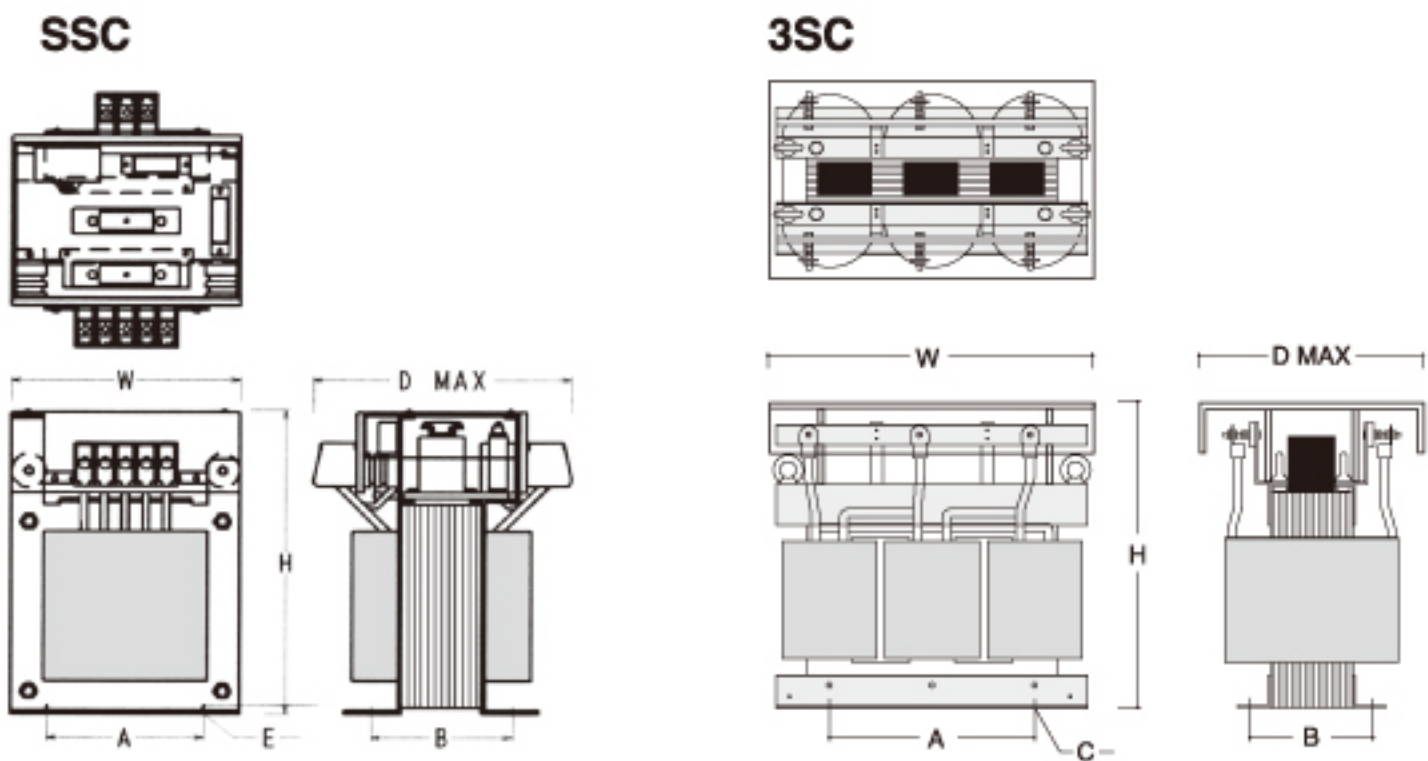
形状・寸法図
