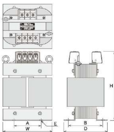
UP形 (ねじアップ式端子台)
