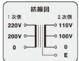
KT形 (端子台)
