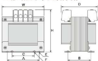
UP形 (ねじアップ式端子台)
