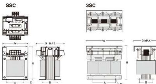
形状・寸法図
