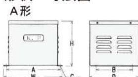
形状・寸法図
